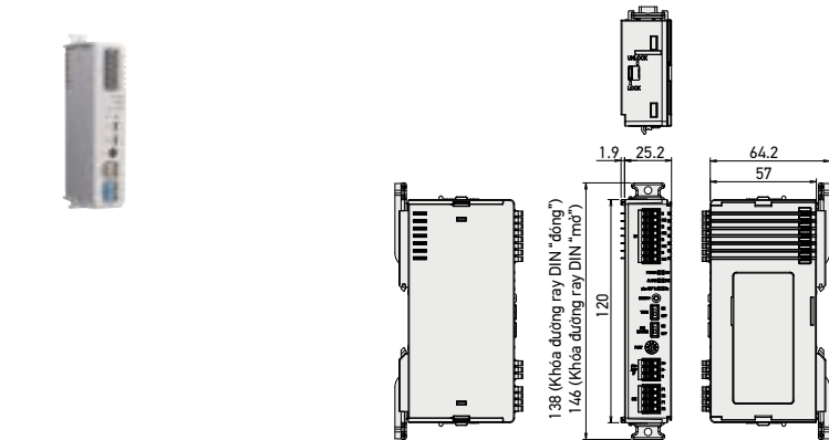
Khe cắm bộ chuyển đổi DIII plus DGE601A53
