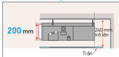
Hình chiếu cạnh
