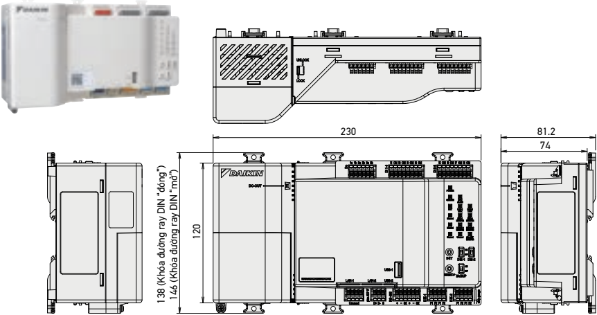
MARUTTO edge DGE601A51
