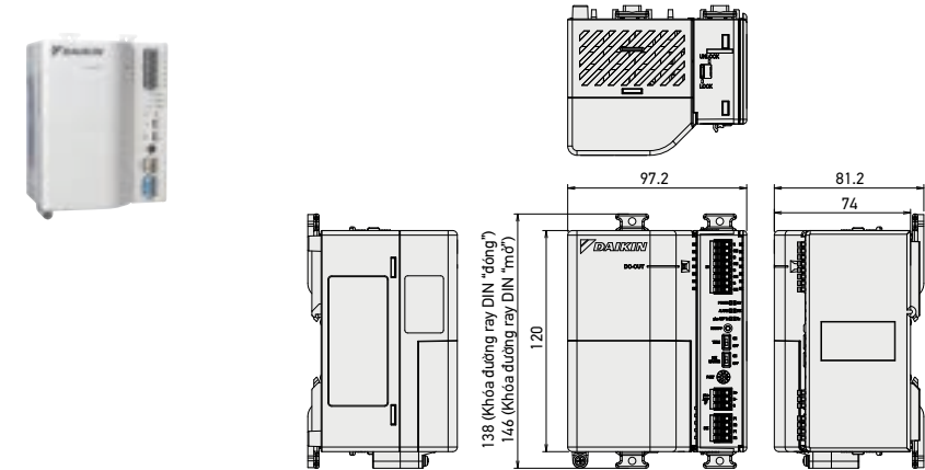
Bộ chuyển đổi DIII plus DGE601A52
