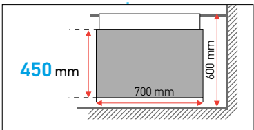
Hình chiếu bằng
